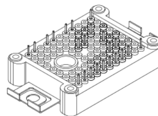
外形示意图
