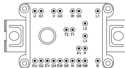
引脚示意图
