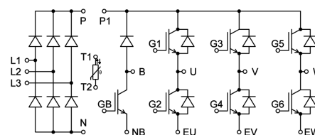
电路示意图
