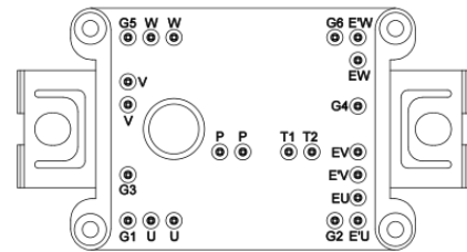
引脚示意图
