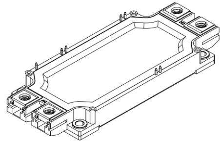
外形示意图
