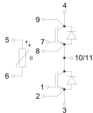
电路示意图
